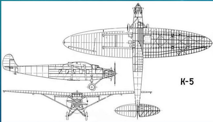
Эскиз безмоторного самолета К 5
